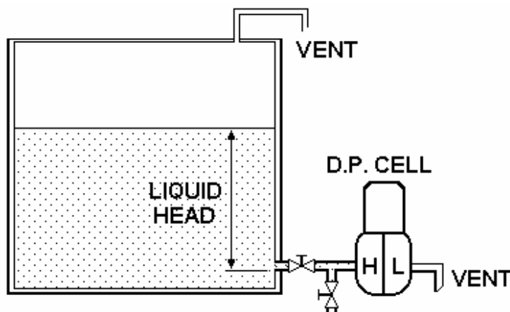
شکل ۴-۲- D.P. cell متصل شده به یک مخزن روباز
